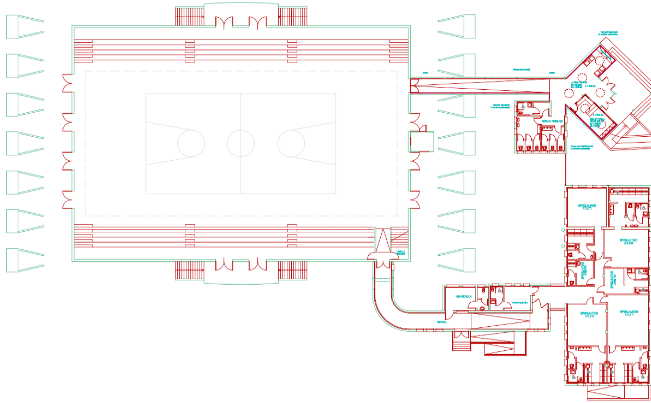
PIANTA PIANO RIALZATO Scala 1:100
